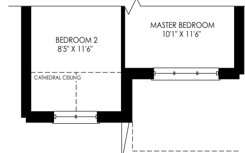
ELEVATION BB
