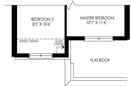
ELEVATION AC
